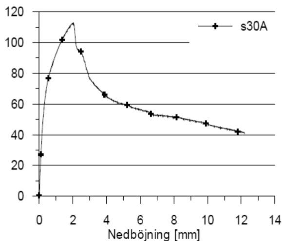
Figur 3.1 Resultat från böjprov i rärläge.
